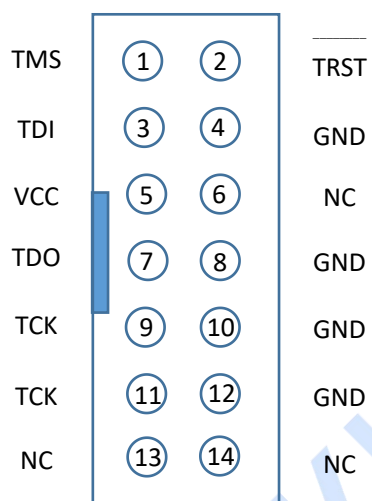
14PIN-JTAG
